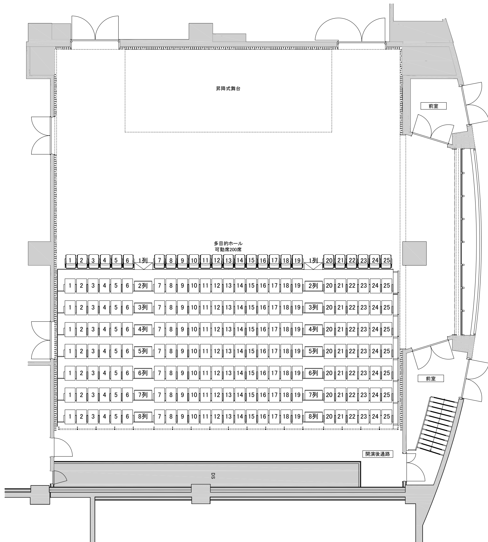
多目的ホール 座席表(B)[可動席] Scale(A3)1:100
